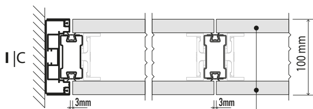
"A-A"
